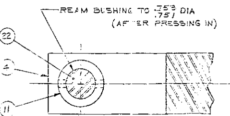
SECTION C-C SCALE: FULL
